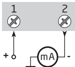
Instalación de 2 hilos
